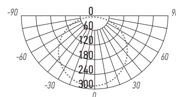
PBH-PC-RA SPEC 18w
